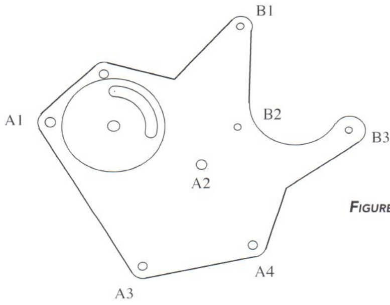
M1 BRACKET
